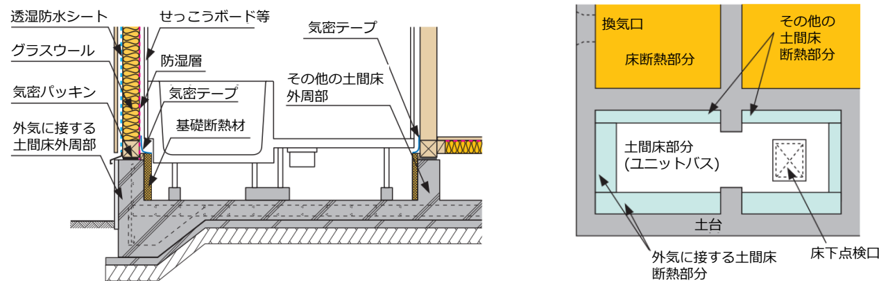
▲ 基礎断熱を行う場合の使用例
