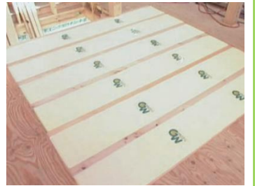
外気に接する床の施工例
